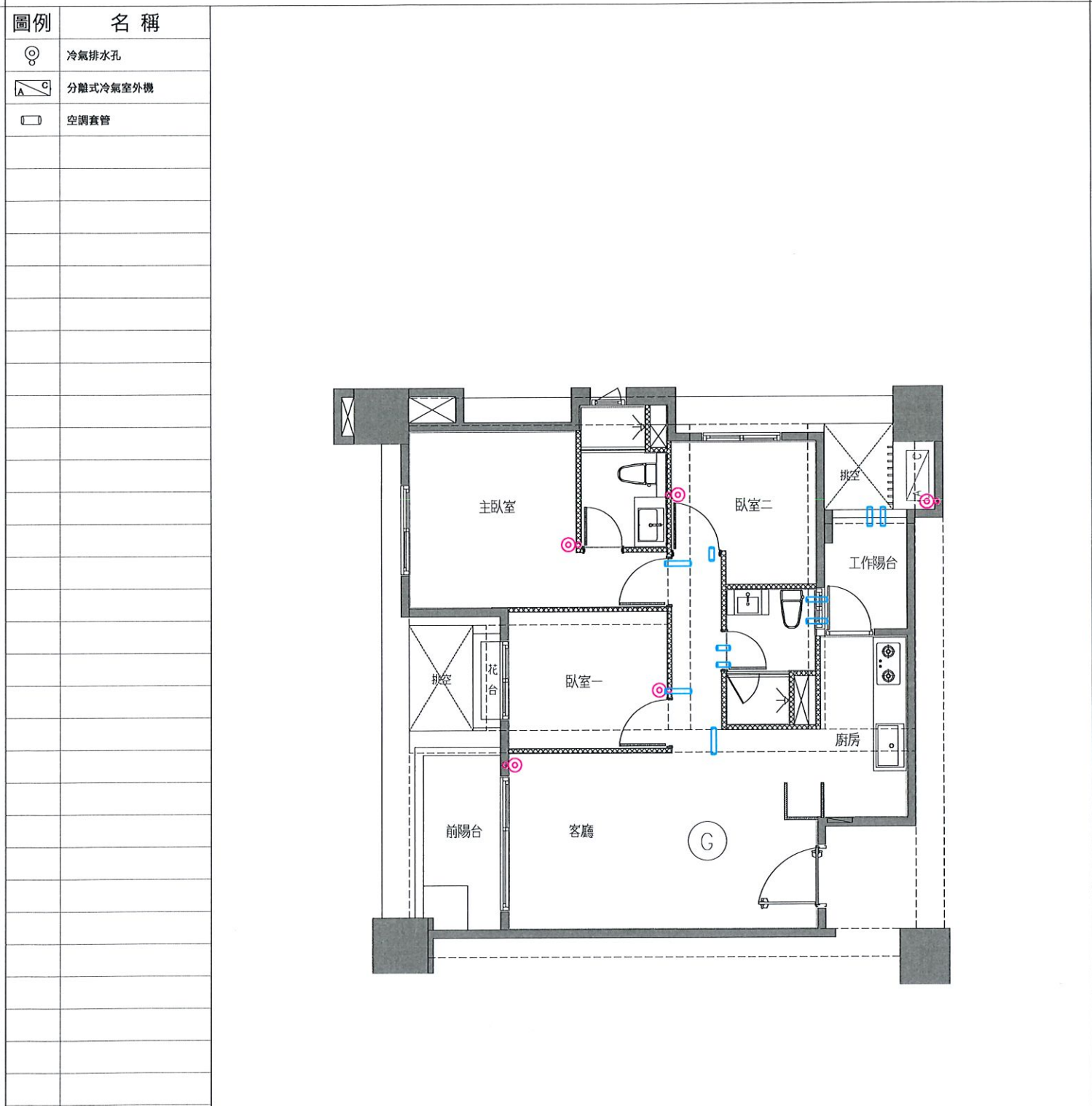
G戶 冷氣套管及排水位置示意圖(套上層樑)
