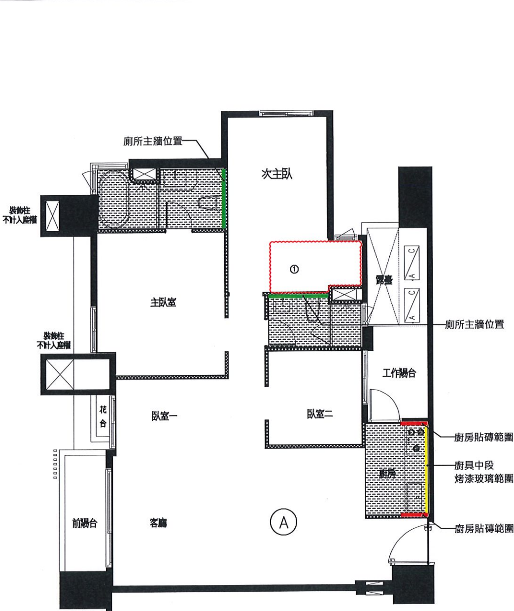
<變更後平面圖>
