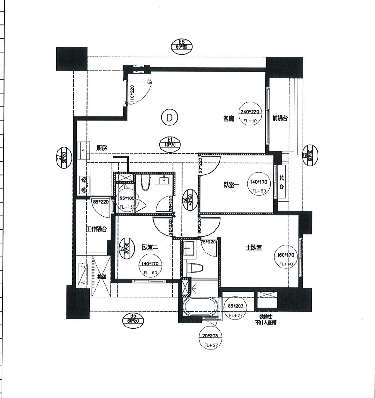
D戶 建築平面圖(套上層樑)
