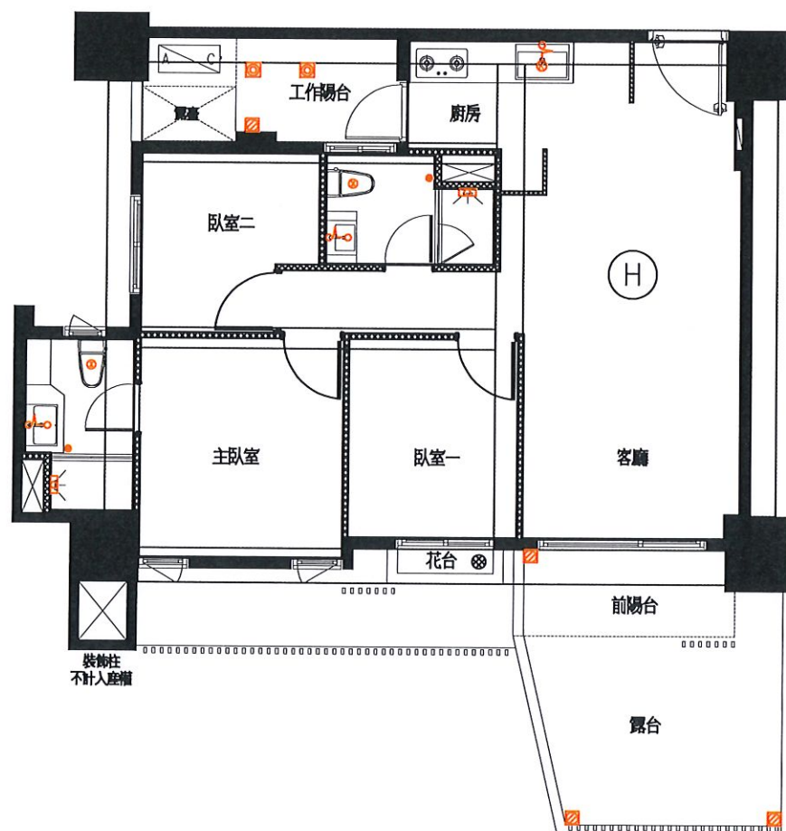
H戶 排水示意平面圖(套下層樑)
