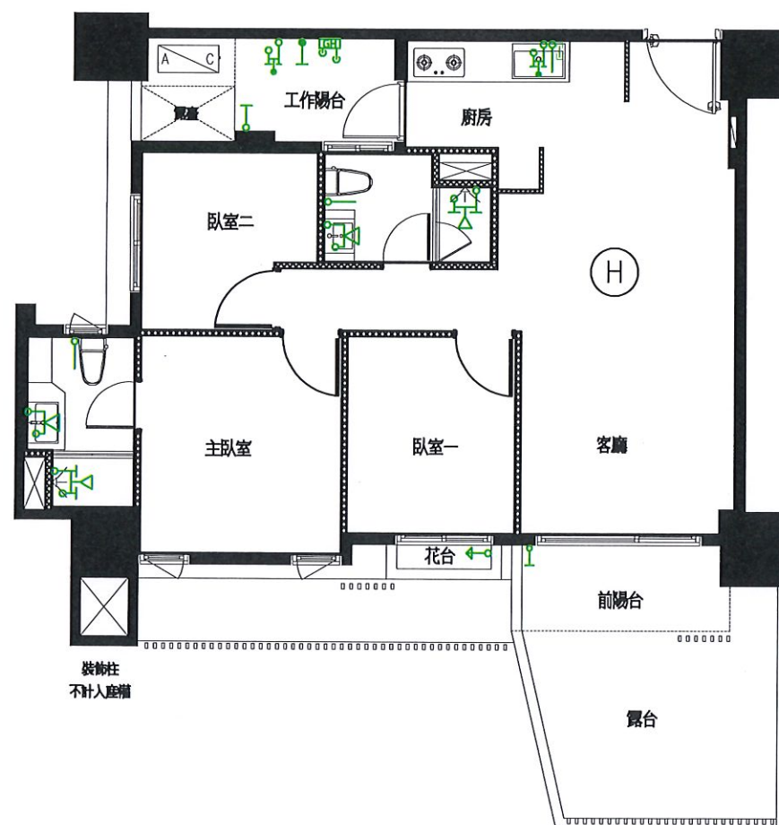
H戶 給水示意平面圖
