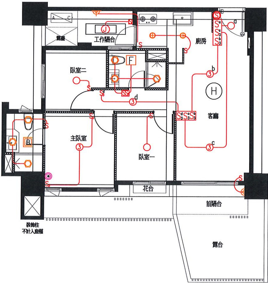
H戶 電燈開關及迴路示意圖(套上層樑)
