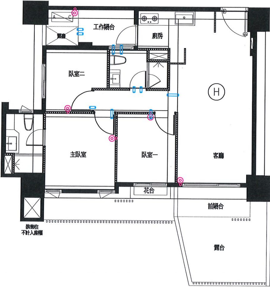
[H戶] 冷氣套管及排水位置示意圖(套上層樑)
