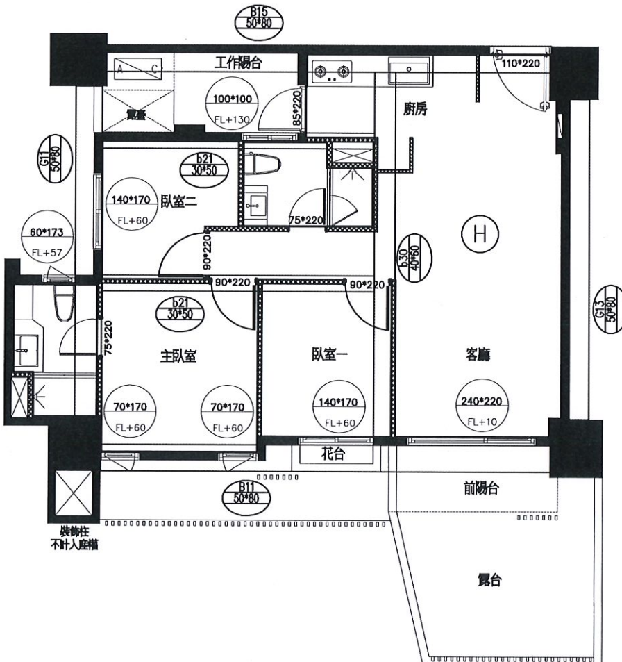
H戶 建築平面圖(套上層樑)
