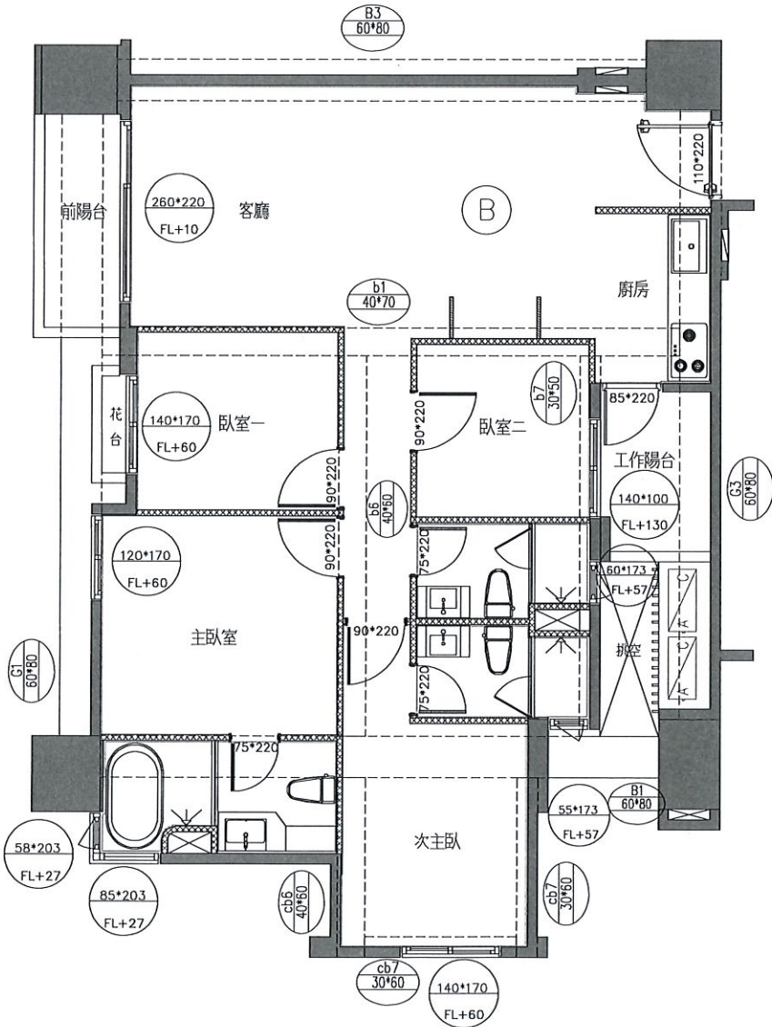
B戶 建築平面圖(套上層樑)
