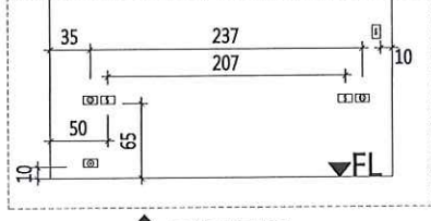
Ⓓ D向立面圖
