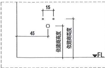
E向立面圖
