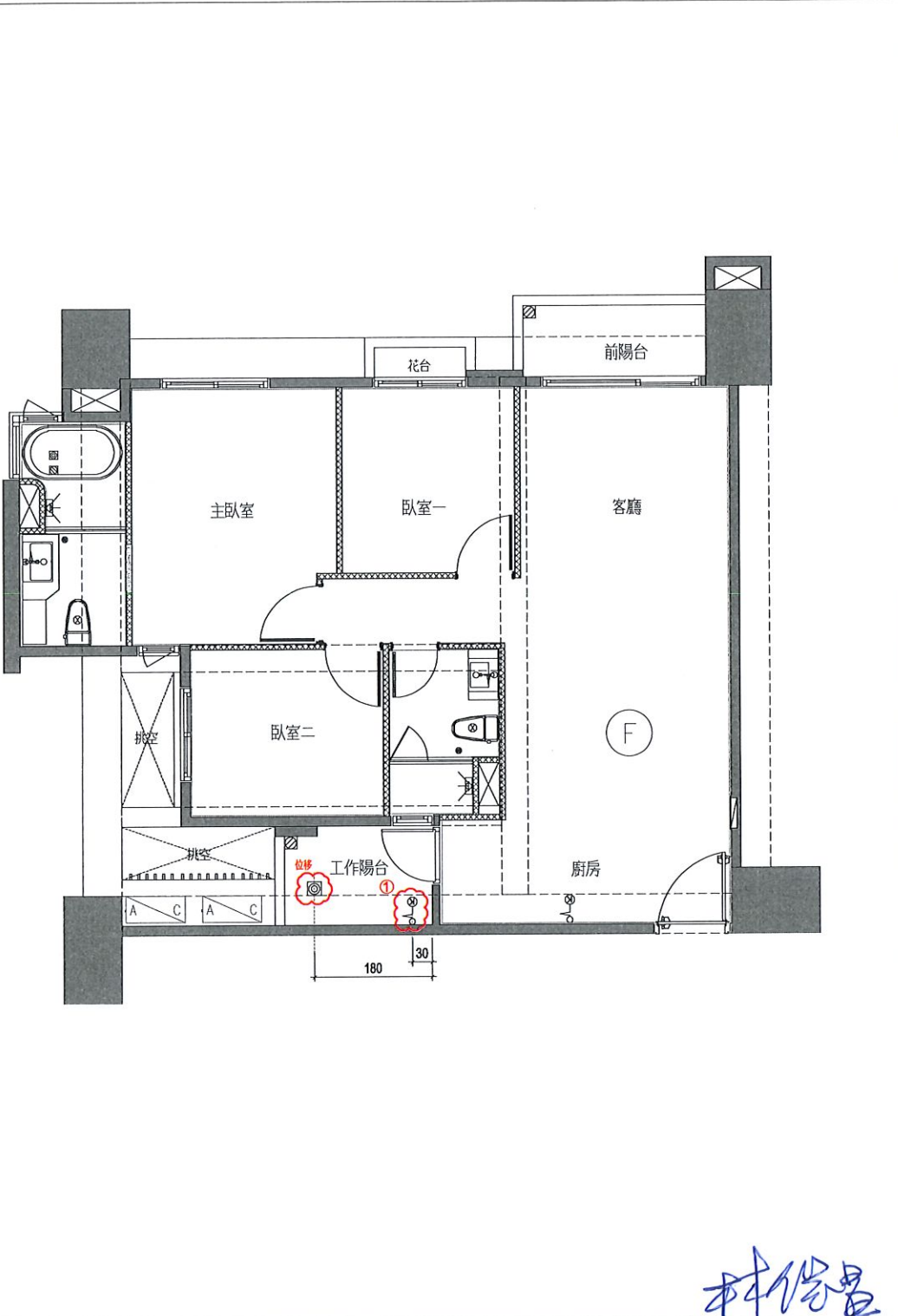
<變更後平面圖>
