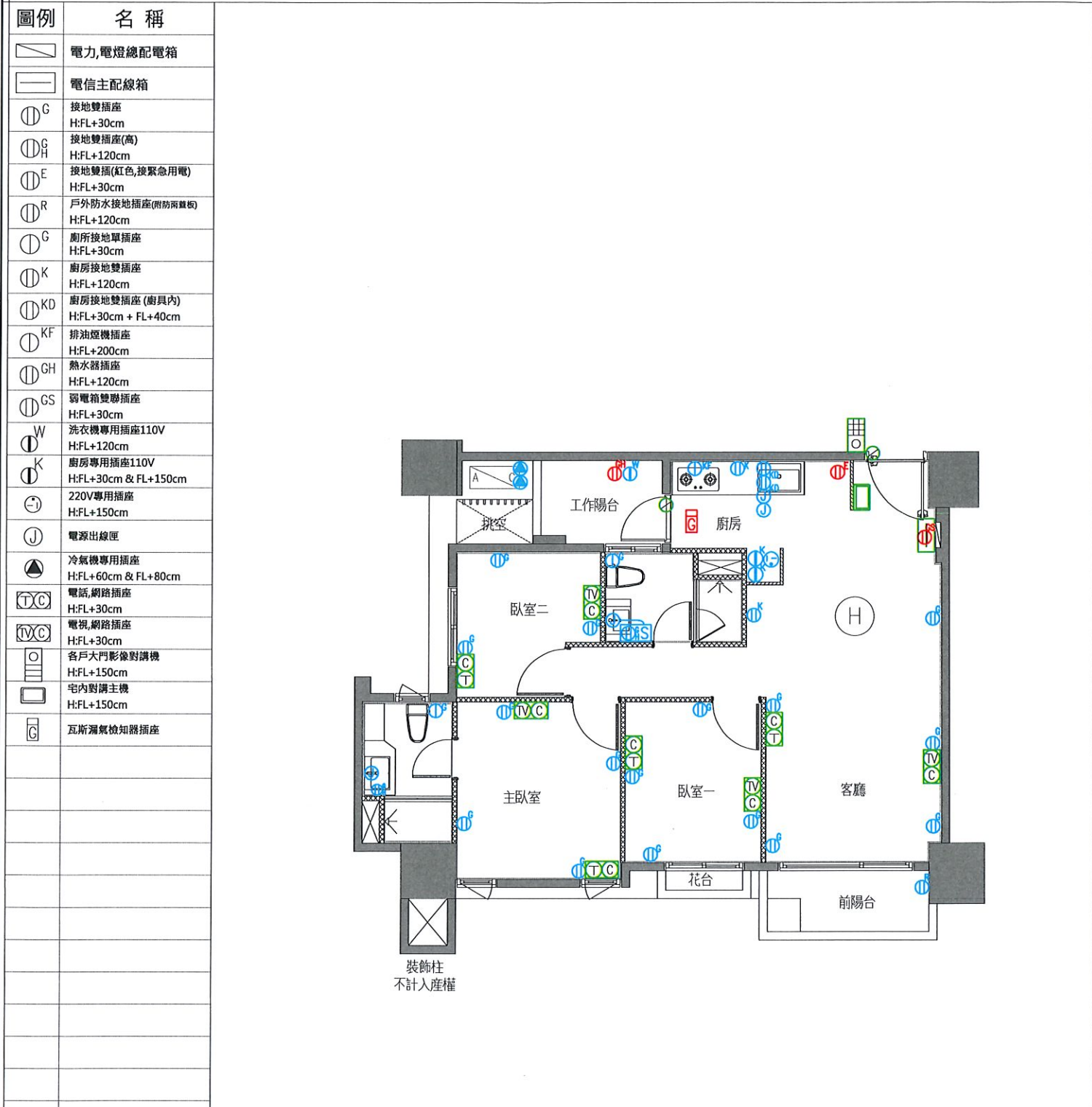
H戶 插座及弱電位置示意平面圖
