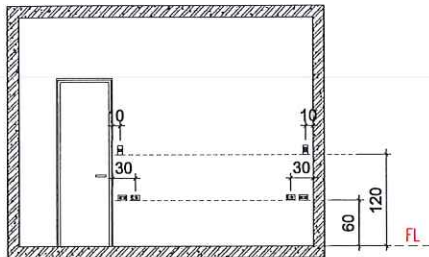
主臥床頭牆插座開關位置
