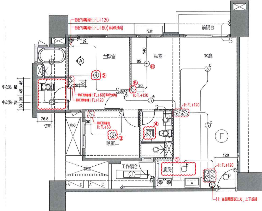
主臥床頭牆插座開關位置
