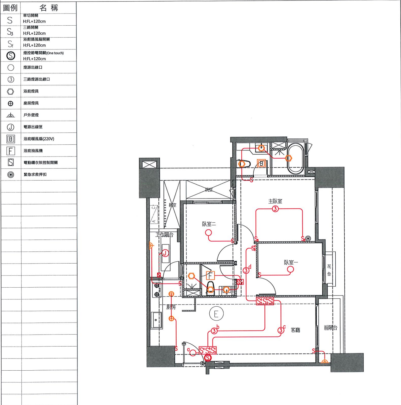
<原設計平面圖>
